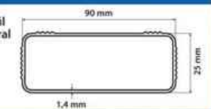
Escada Elite 90 c/ Corda (Perfil Lateral 90mm)
