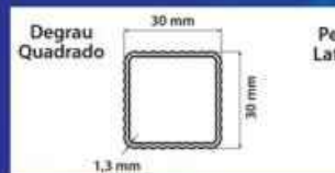
Escada Degrau Quadrado Super (Perfil L. 80mm)
