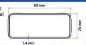
Escada Degrau Quadrado Super c/ Corda (Perfil L. 80mm)
